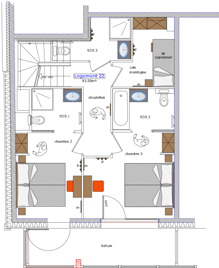
Plan du Logement 22 - niveau inférieur R+1
