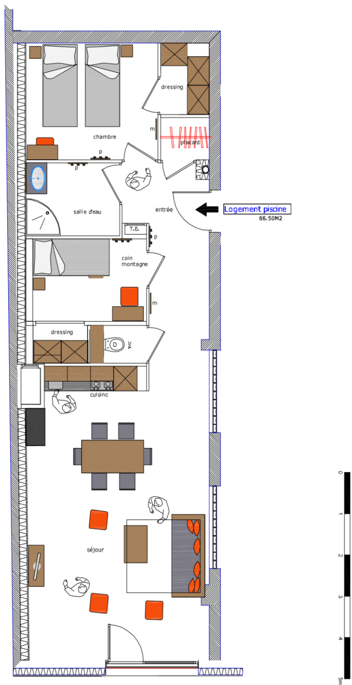
Plan du Logement Piscine - niveau R-2
